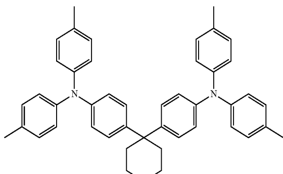
TAPC
