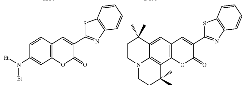
Coumarin 6
