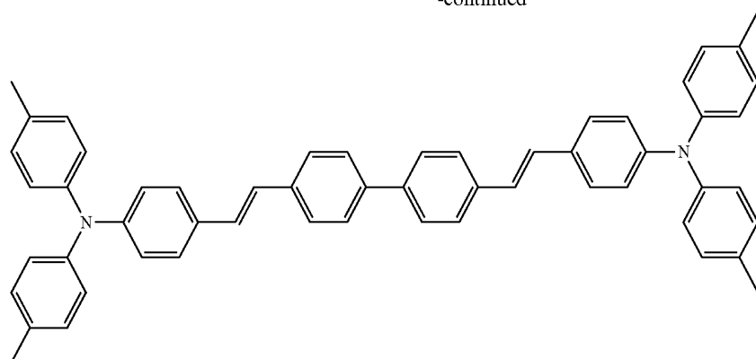
DPAVBi
